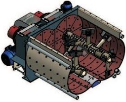
TWIN-SHAFT MİKSER
