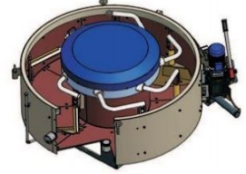
PAN MİKSER
